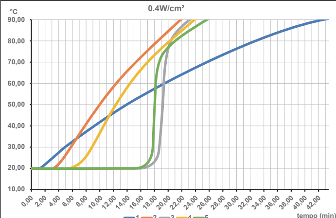
Con un carico superficiale di 0.4W/cm 2 (240W)
