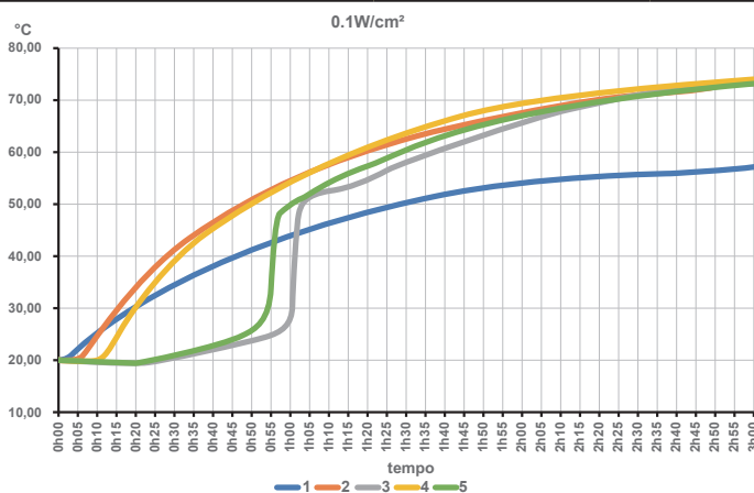
Con un carico superficiale di 0.1W/cm 2 (60W)
