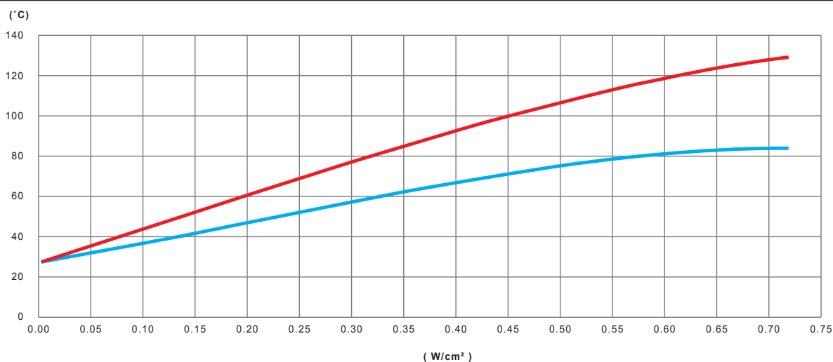
Variazione, in funzione della potenza in W/cm² del nastro riscaldante in silicone, della temperatura della parete di un tubo in PVC riempito con acqua non circolante, non isolato termicamente.
